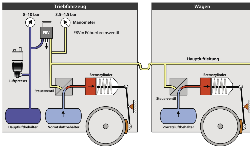
Abb. 2-8: Funktionsprinzip der indirekt wirkenden selbsttätigen Druckluftbremse – Bremsstellung
